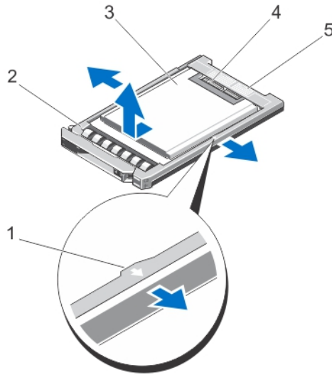
Abbildung 22. Entfernen und Installieren eines 1,8-Zoll-SSD-Laufwerks aus einem/in einem SSD-Laufwerksträger
