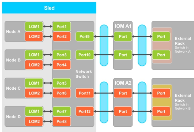
Abbildung 7. Isolierte Netzwerk-Konfiguration
