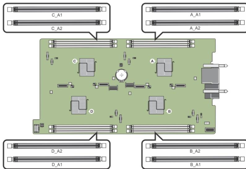
Abbildung 13. Positionen der Speichersockel
