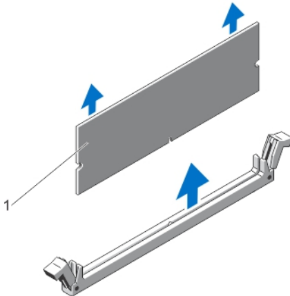
Abbildung 15. Entfernen des Speichermoduls
