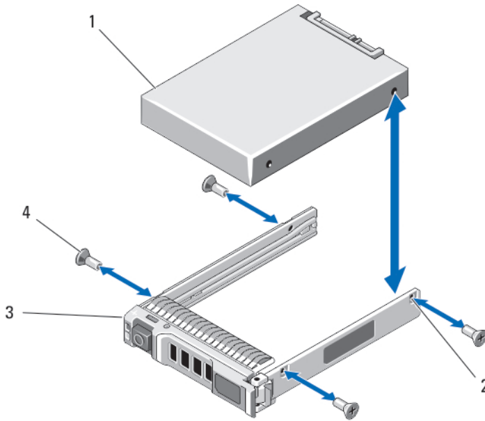
Abbildung 21. Entfernen und Installieren eines 2,5-Zoll-Festplatten-/SSD-Laufwerks aus einem/in einem Festplatten-/SSD-Laufwerksträger
