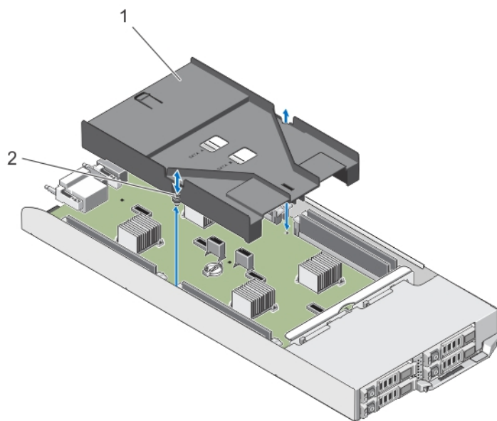
Abbildung 12. Entfernen und Einsetzen des Kühlgehäuses
