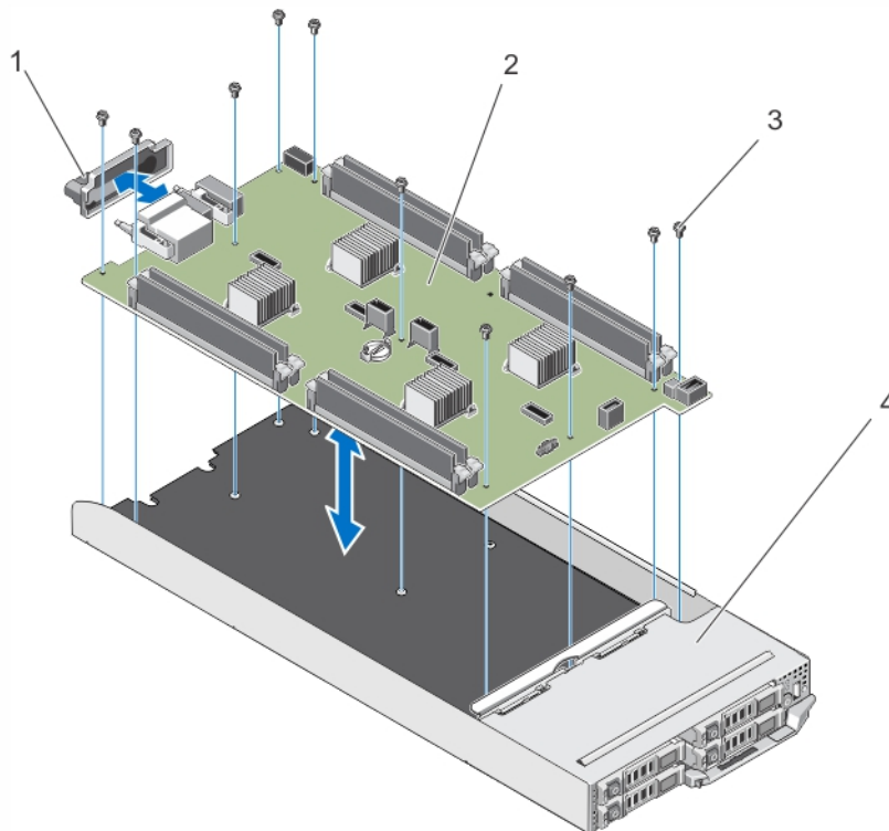
Abbildung 27. Entfernen und Einsetzen der Systemplatine
