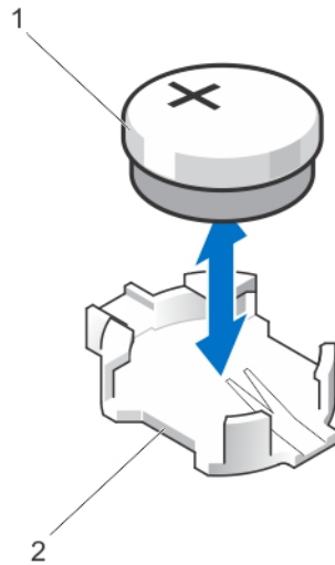
Abbildung 26. Austauschen der Systembatterie
