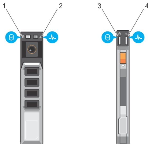
Abbildung 3. Festplatten-/SSD-Laufwerksanzeigen
