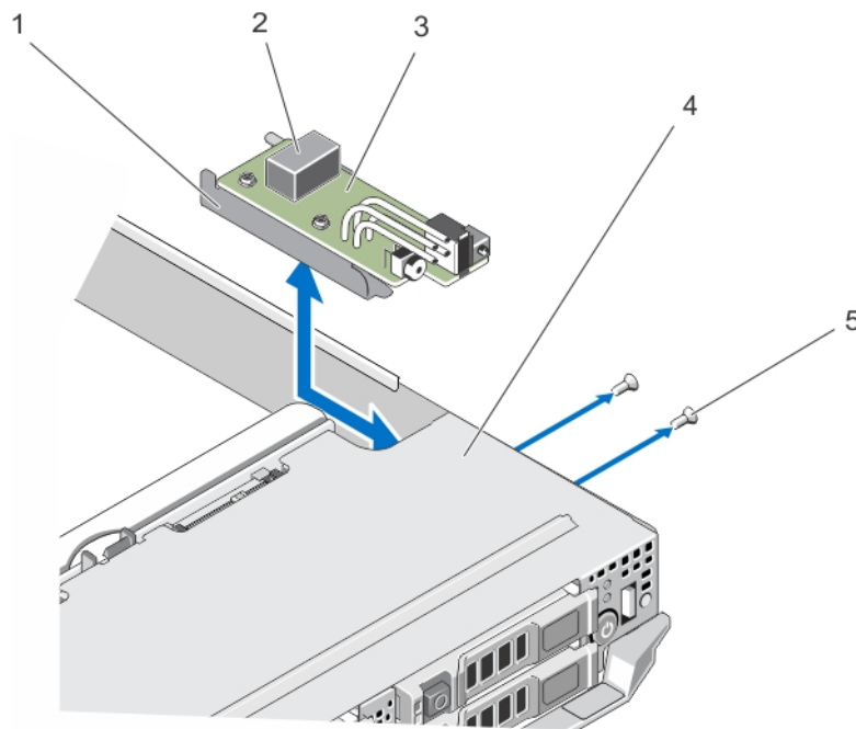
Abbildung 28. Entfernen und Installieren des Bedienfelds
