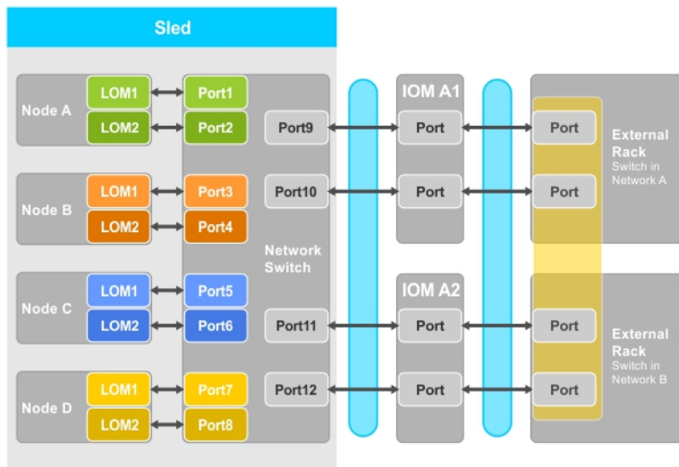
Abbildung 6. Netzwerkadapter-Isolationskonfiguration
