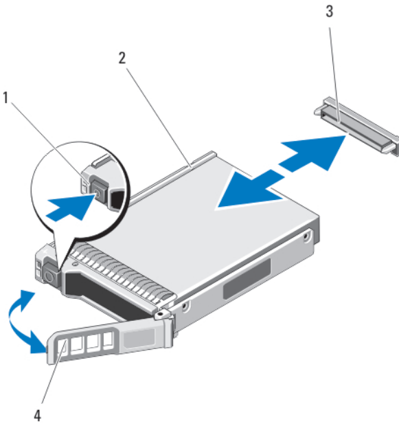
Abbildung 19. Entfernen und Installieren eines 2,5-Zoll-Festplatten-/SSD-Laufwerks
