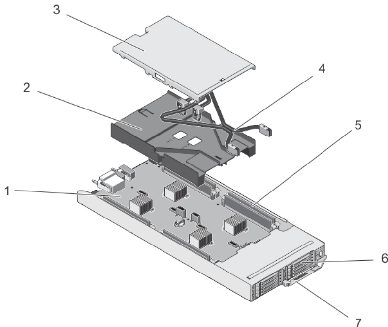
Abbildung 10. Das Innere des Schlittens – 1,8-Zoll-SSD-System
