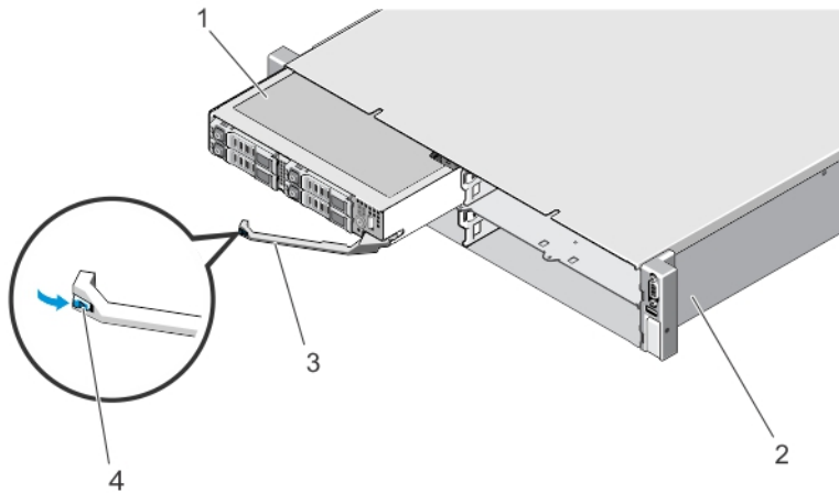
Abbildung 8. Entfernen und Installieren eines Schlittens
