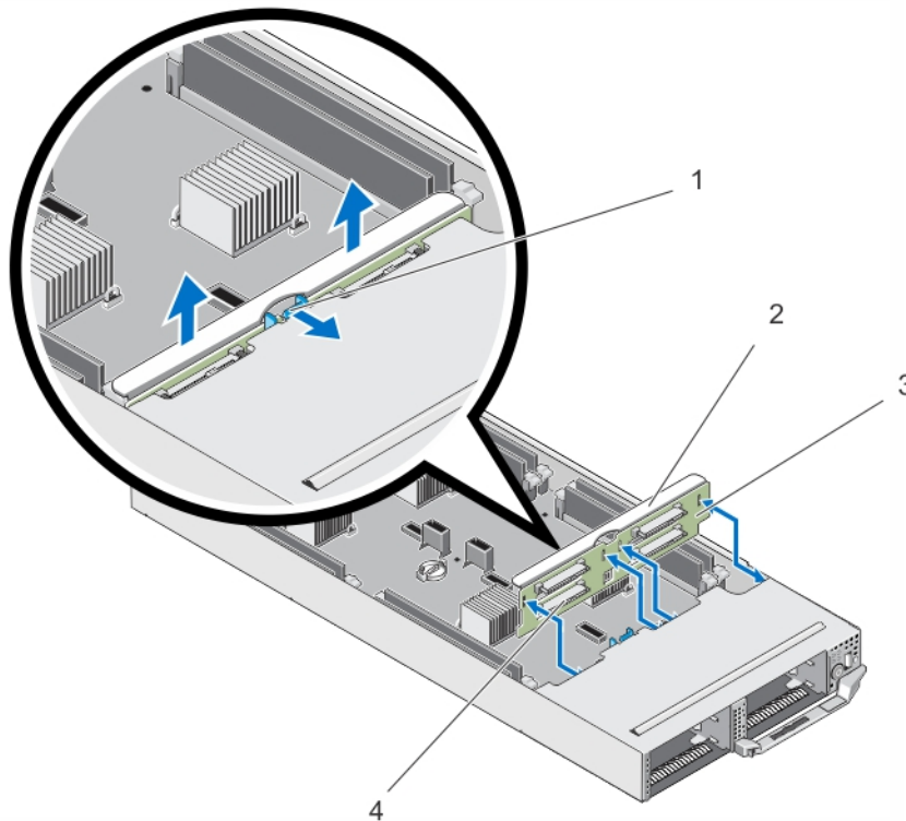
Abbildung 23. Entfernen und Installieren der Festplatten-/SSD-Rückwandplatine
