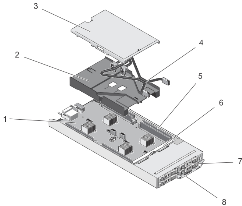
Abbildung 9. Das Innere des Schlittens – 2,5-Zoll-Festplatten-/SSD-System
