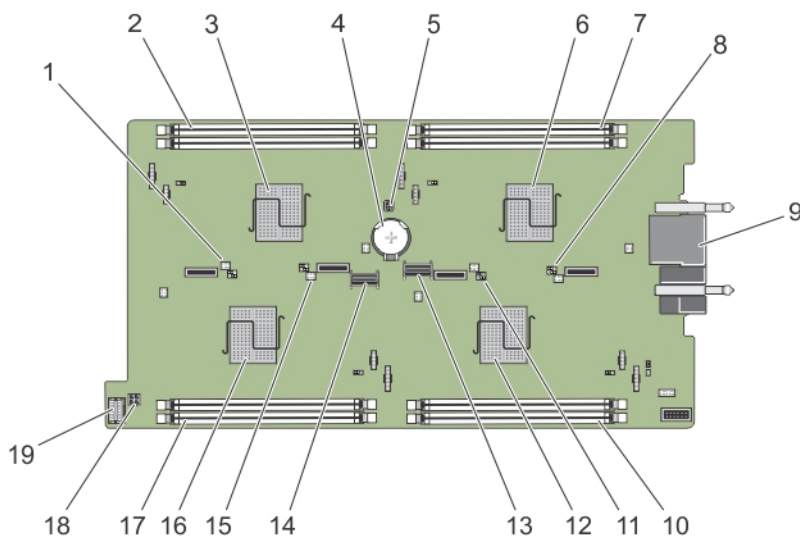
Abbildung 29. Systemplattenanschlüsse
