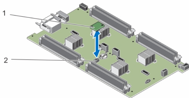
Abbildung 25. Austauschen der ERM
